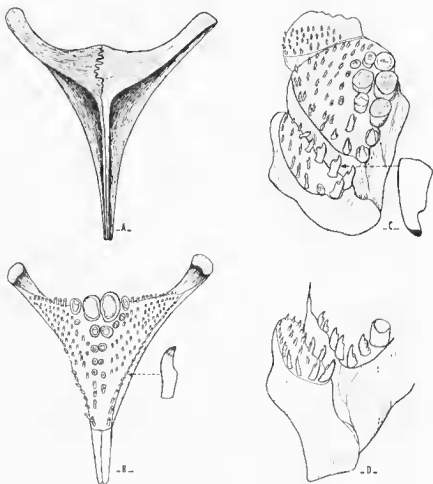
FIG. 11. — Paretroplus kieneri Arnoult. A : Pharyngien inférieur, face interne et symphyse. B : Pharyngien inférieur, face externe. C : Pharyngien supérieur, vue de dessus. D : Vue de 3/4 avant.
